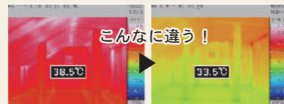
一般の断熱工法 冷房を使用しない部屋の小屋裏温度を測定(8月末)
